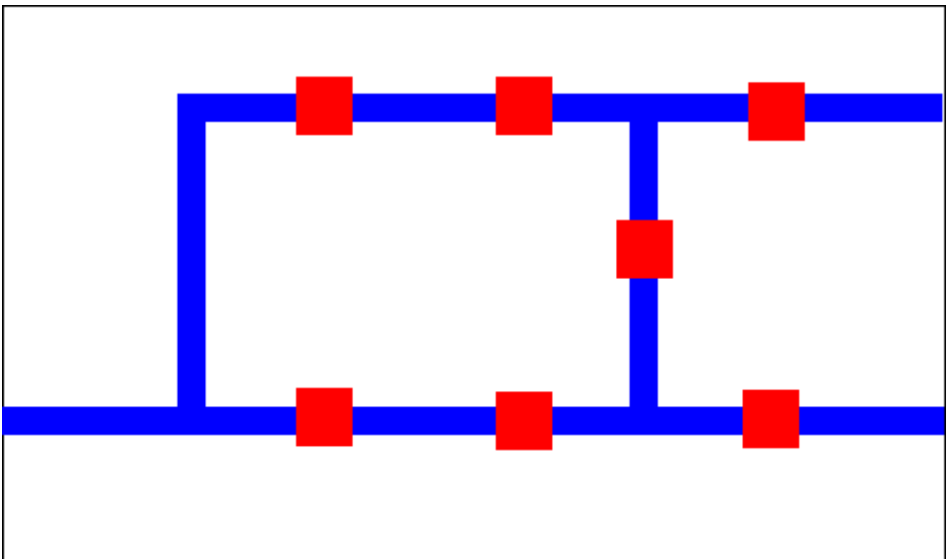
SCHEMATISIERTER STADTPLAN VON KÖNIGSBERG
