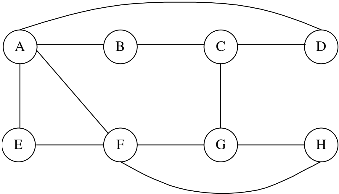
GRAPH, IN DEM ZWAR KEIN EULERKREIS, ABER EIN EULERWEG EXISTIERT
