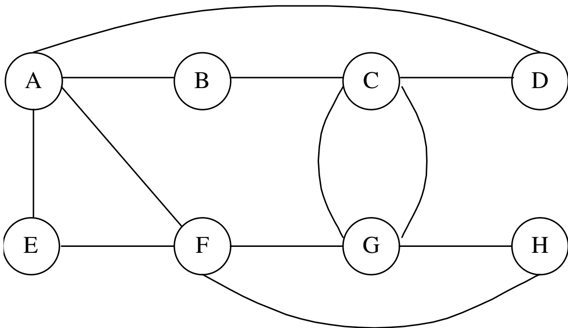
GRAPH, IN DEM EIN EULERKREIS EXISITERT
