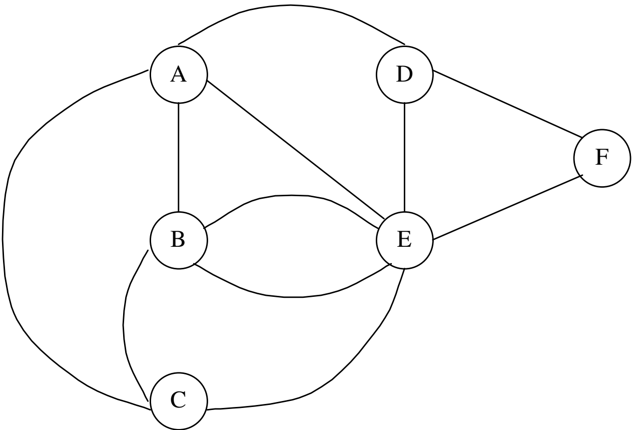
GRAPH, IN DEM EIN EULERWEG EXISTIERT
