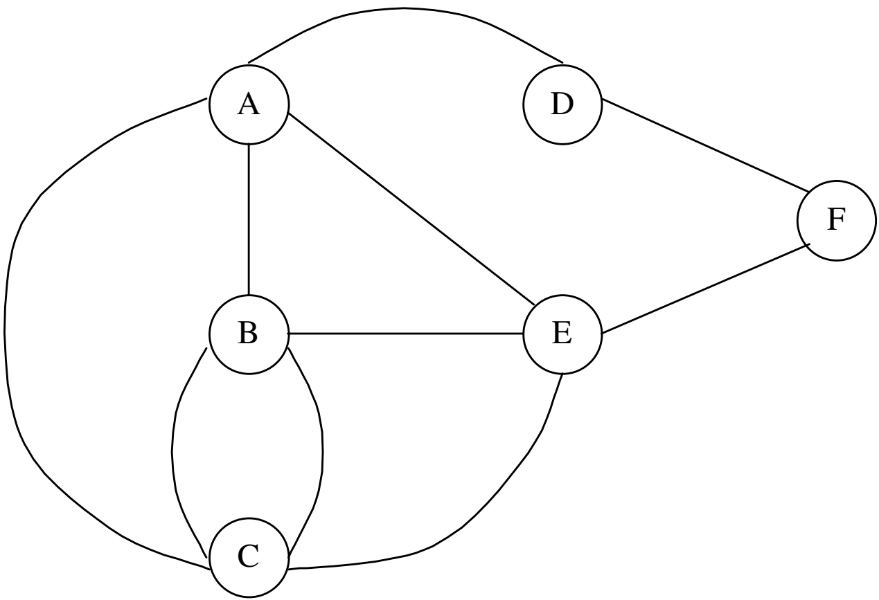
GRAPH, IN DEM EIN EULERKREIS EXISITERT
